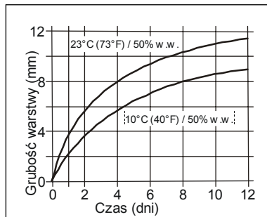
Szybkość utwardzania Sikaflex 252
